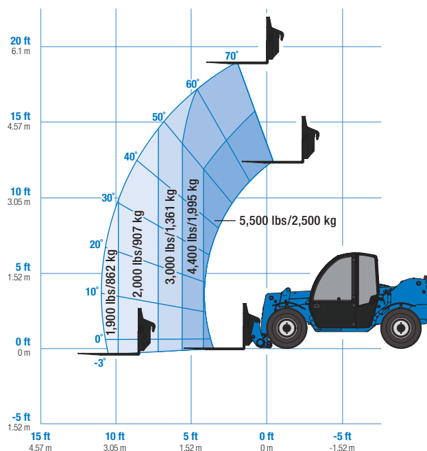
Gráfico de Carga del GTH™ -5519
