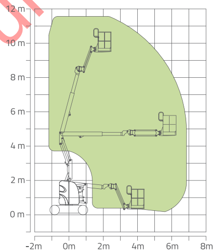
Curva de amplitud de plataforma ZA10RJE
