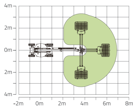
Curva de amplitud de plataforma ZA10RJE
